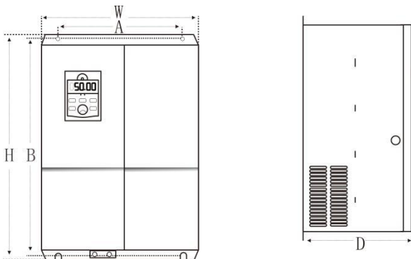
5.5-160kw外观尺寸
