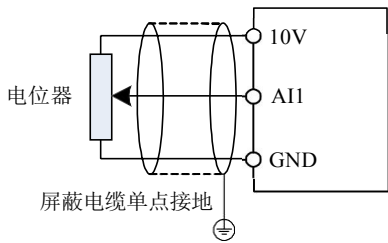
图 3-5. 模拟量输入端子接线示意图
