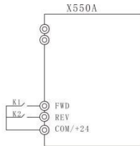
图5-1两线式运转模式1
